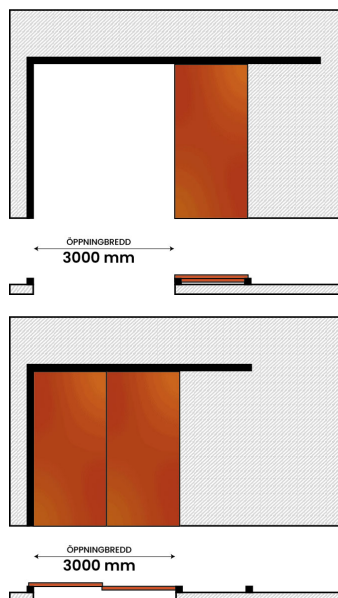
Enkelflyglig teleskoperande
