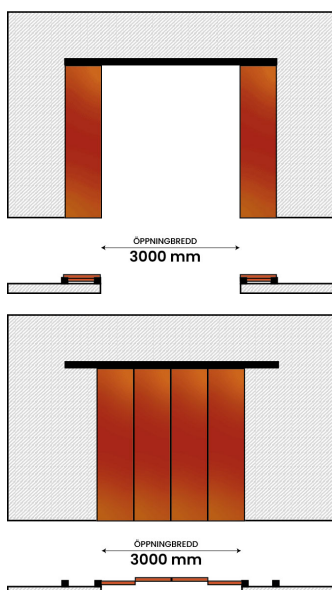
Dubbelflyglig teleskoperande
